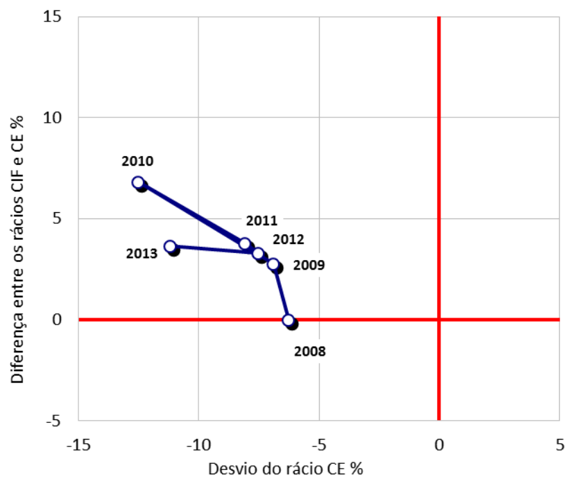
Figura 2.1.3 – Trajetória de relação entre a diferença rácio CIF - rácio CE (%) e o desvio do rácio CE (%) em Matemática no 3º ciclo – 2008 a 2013
