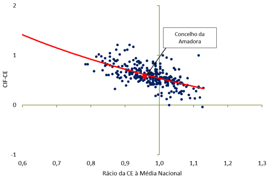
Figura 2.1.2 – Rácio CE e diferença CIF-CE em Português no 2º ciclo – 2013
